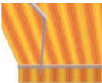
Dessin 2773 PG 1
